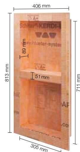
KB 12 N 305 711 A1 s variabilní polici
